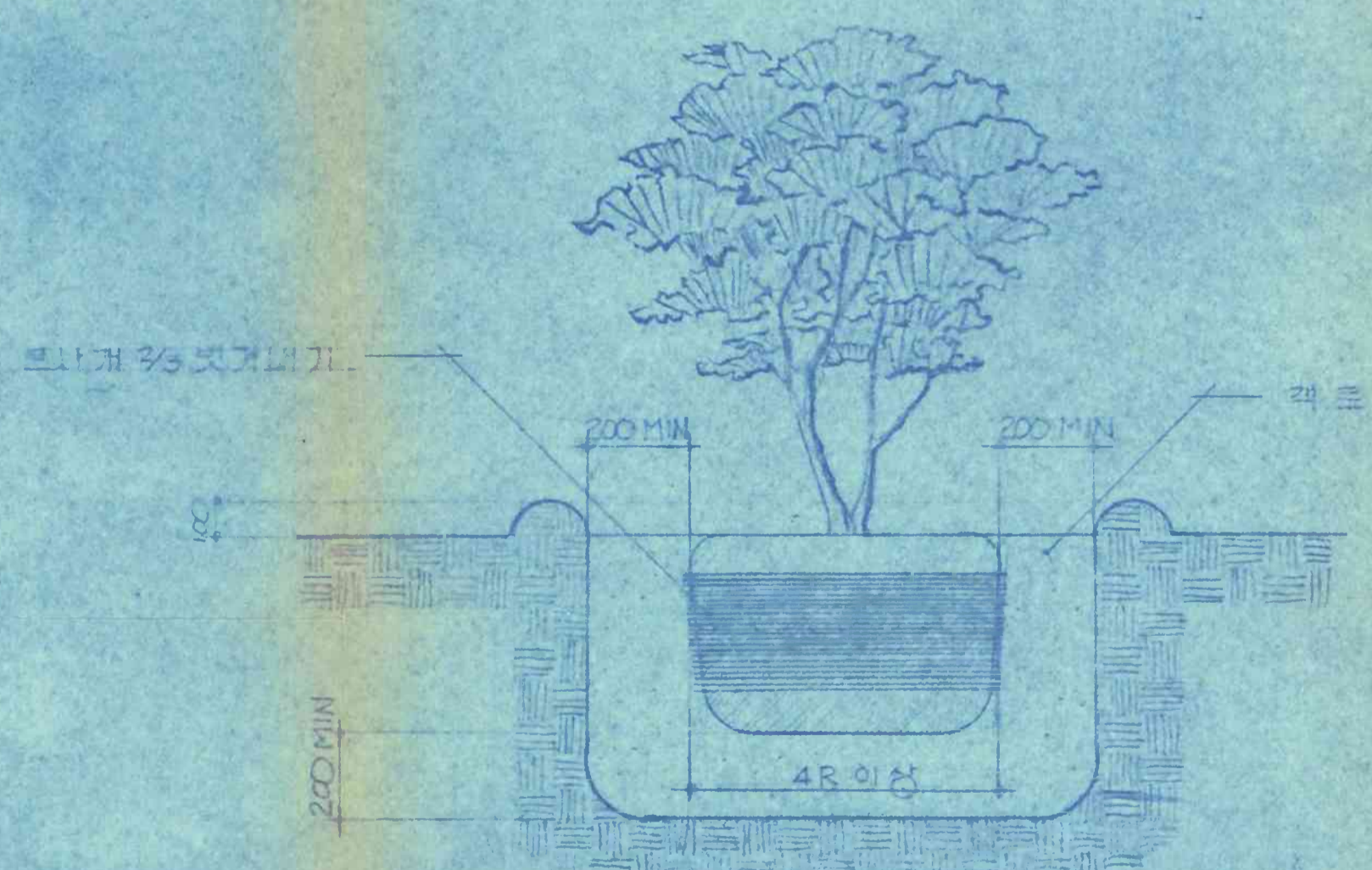
○ H1.0 이상 교목류 식재 상세도
