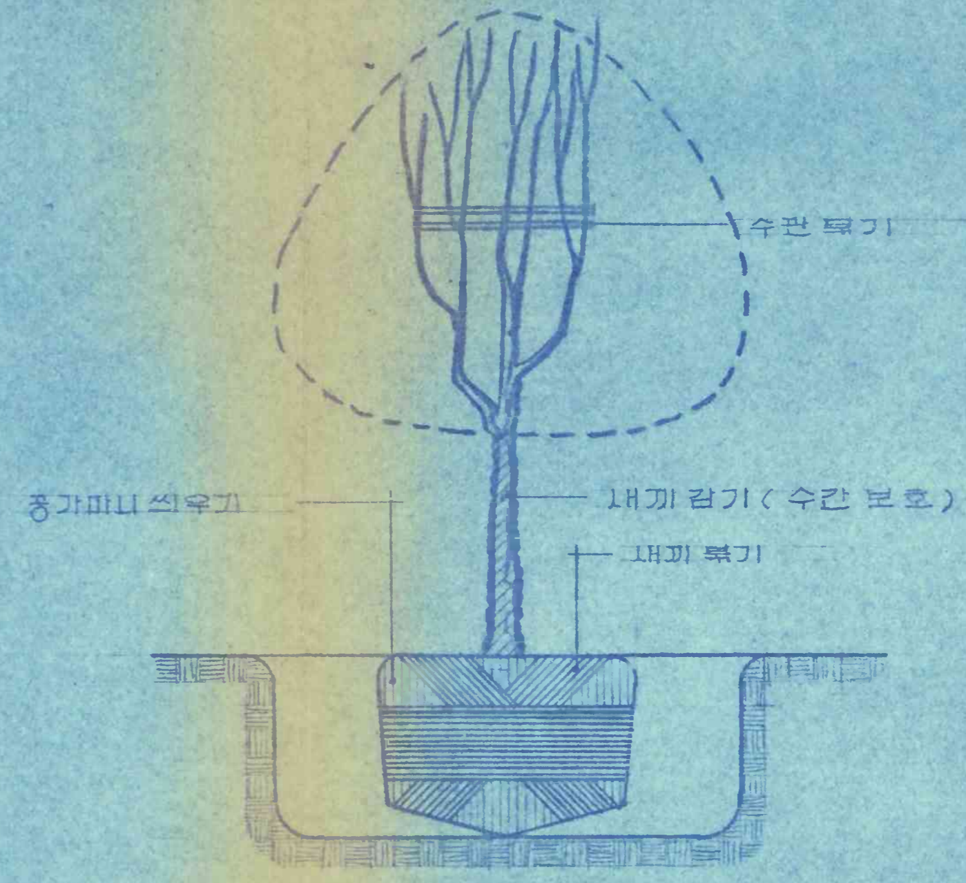
B' TYPE (소형 교목)
