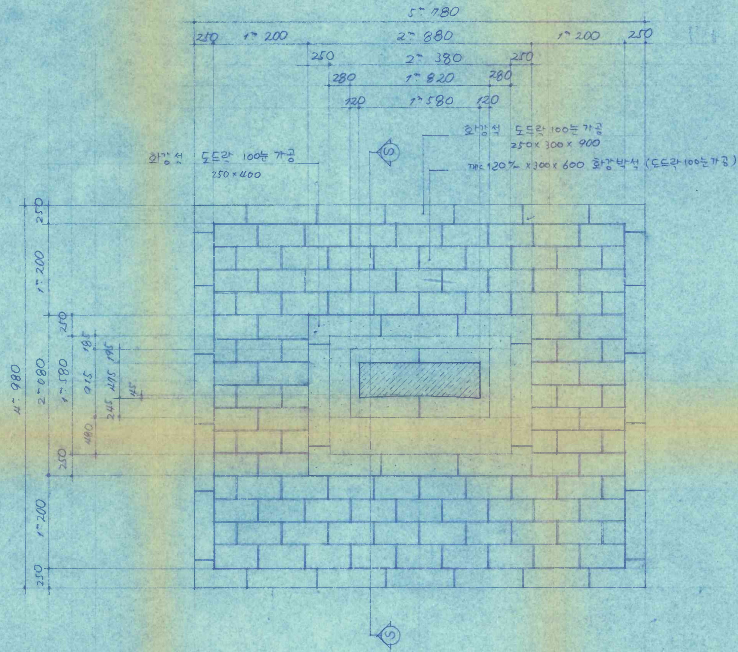
어머니 현장비 평면 상세도 축척: 1/30
