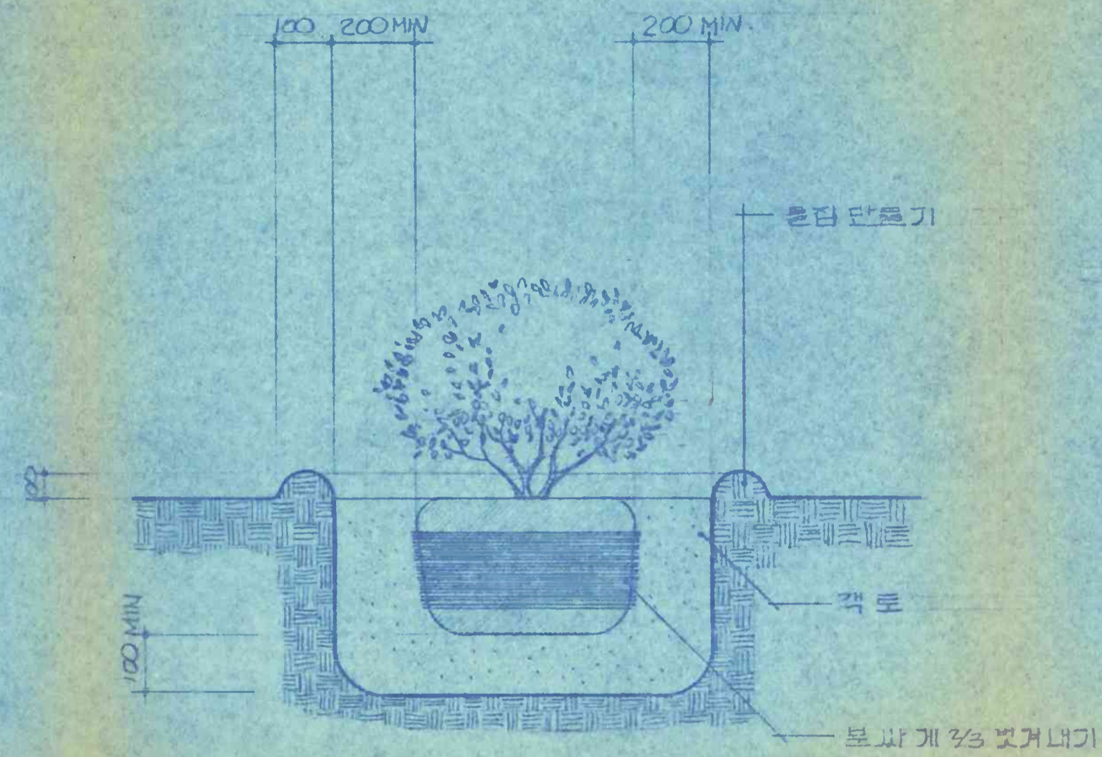
○ H1.0 이하 관목류 식재 상세도
