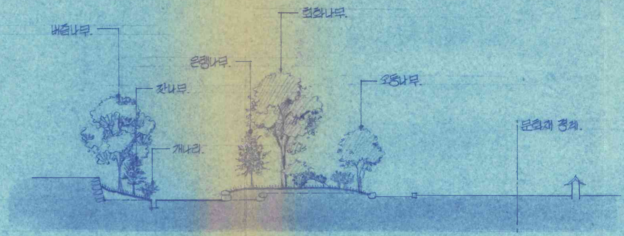
2 +60 화단 단면도 축척 1/300
