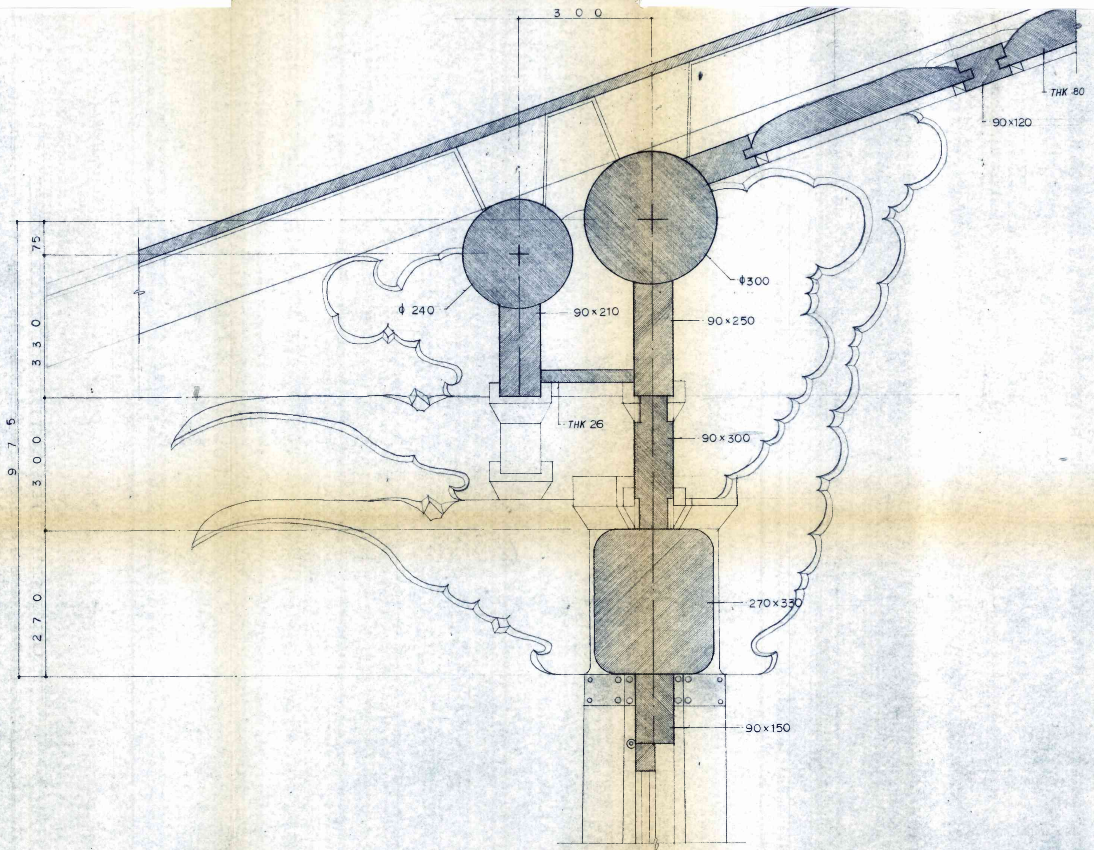
3층 이익공 상세도 SCALE = 1/5
