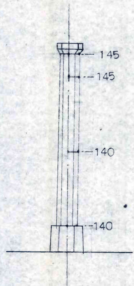
② 번 기둥 기울기 상세도
