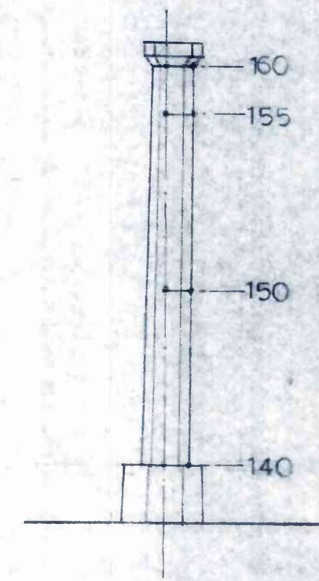
⑦ 번 기둥 기울기 상세도
