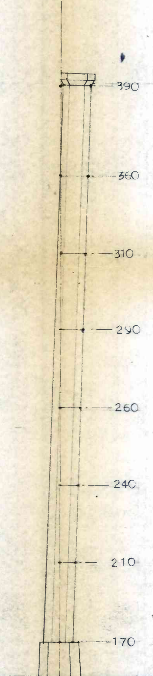
⑤ 번 기둥 기둥기 상세도
