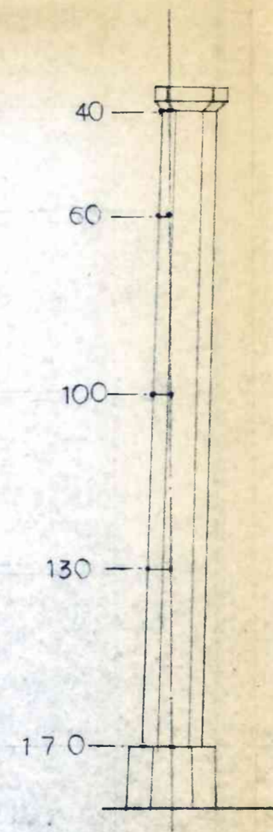
⑤ 번 기둥 기둥기 상세도
