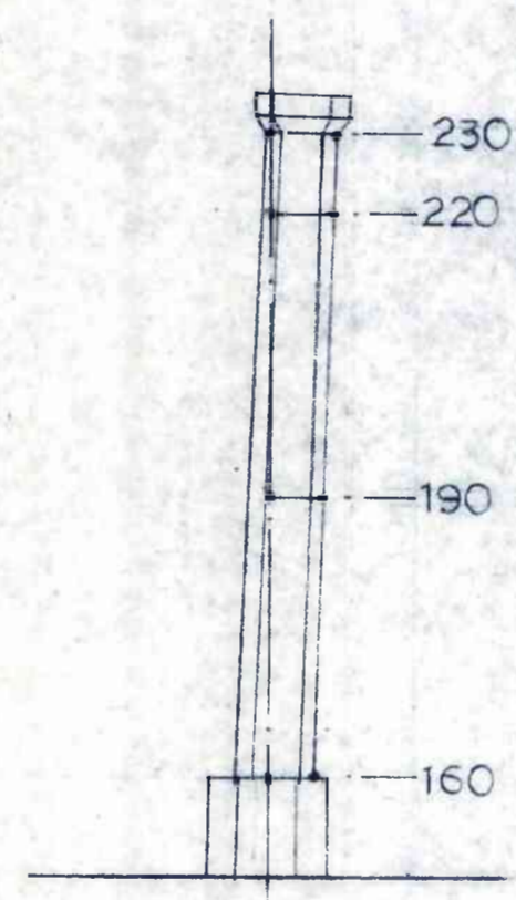
④ 번 기둥 기울기 상세도
