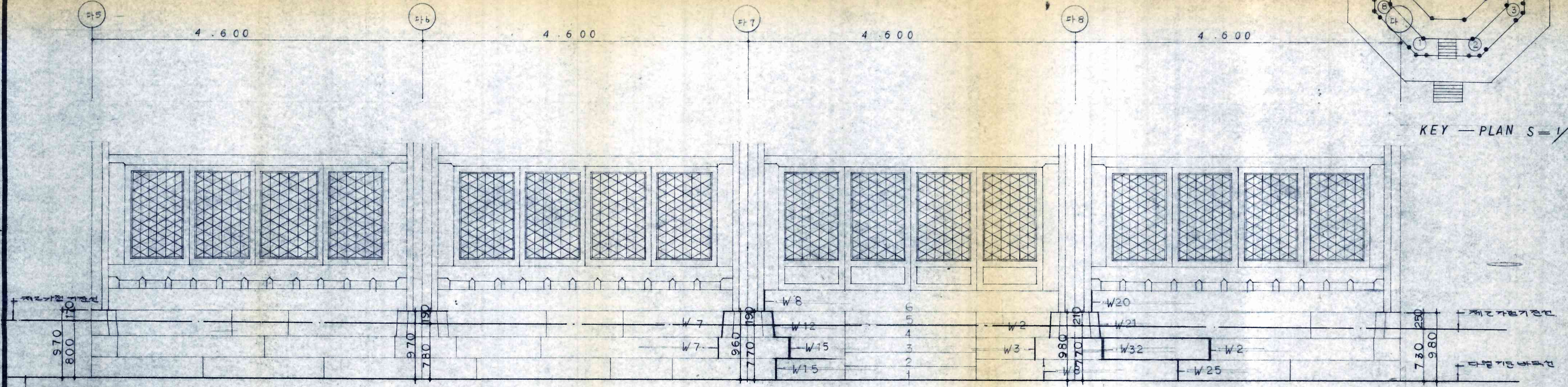
다열 기단 및 창호 전 개도 (변형) SCALE = 1/30
