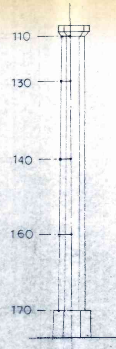
⑧ 번 기둥 기둥기 상세도
