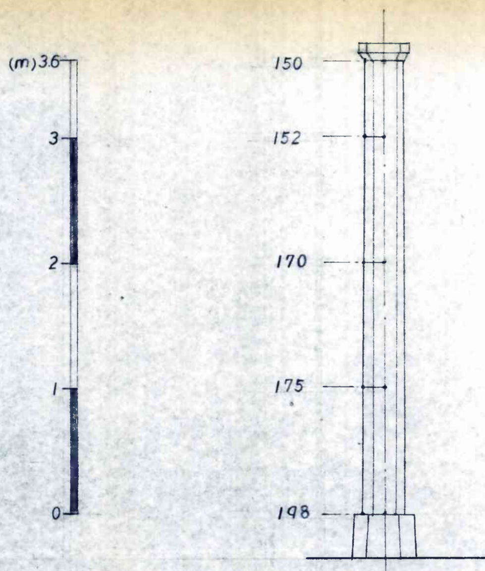
② 번 기둥 기둥기 상세도
