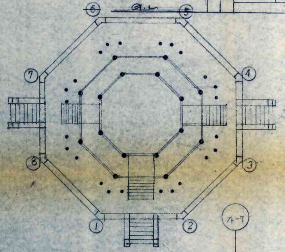
제기일기단 KEY PLAN 1/200
