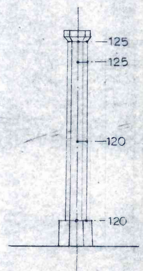
⑧ 번 기둥 기울기 상세도
